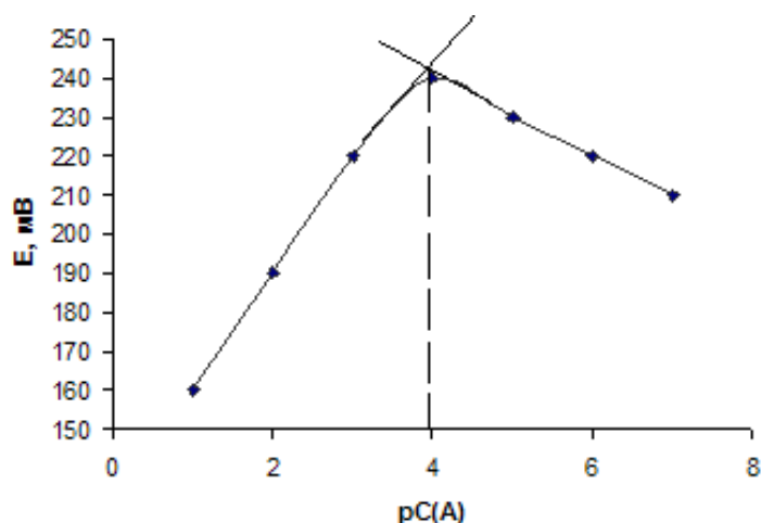
Рисунок 6 - Калибровочная кривая в присутствии постороннего иона
